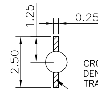
DATIAL B(5:1) TOLERANCE ±0.10)
