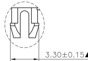
DETAIL A 2:1
